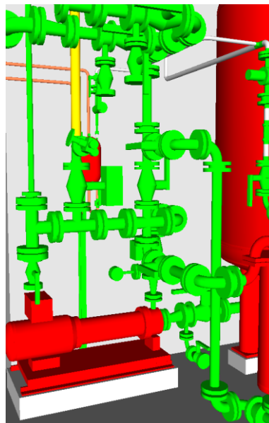
3D 模型
