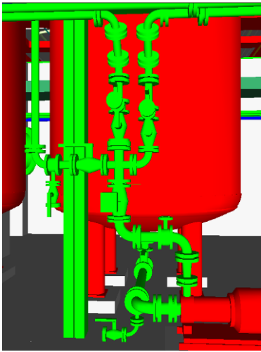
3D 模型
